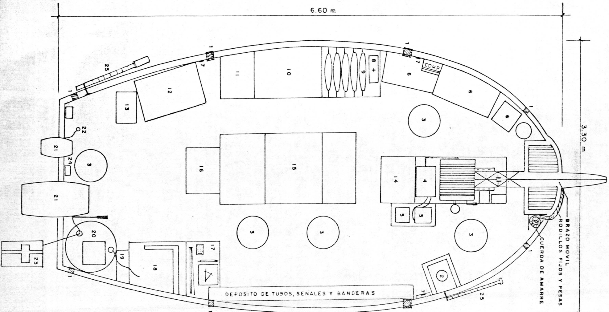
GRAFICO Nº 1 DISTRIBUCION DE EQUIPO EN EL BOTE FLUVIAL PROPUESTO PARA MEDICIONES EN RIOS GRANDES
