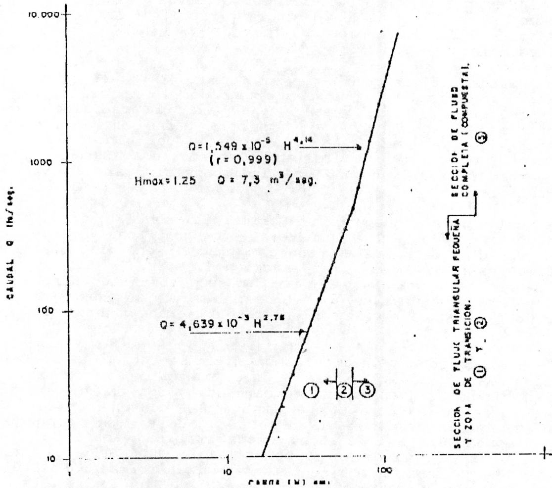
GRAFICO Nº 4 Relación carga-gasto en el prototipo vertedero en el torrente, La Virgen en el Concey.
