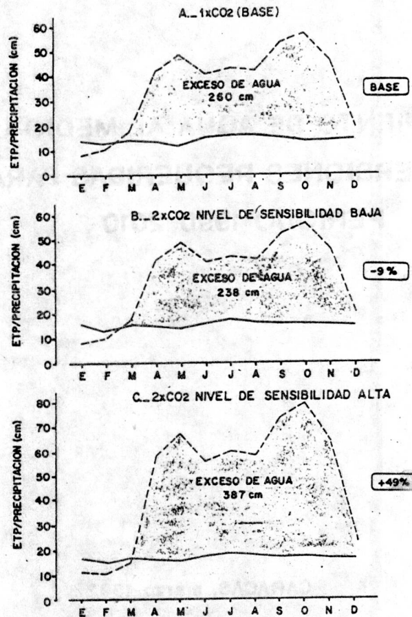
FIG. 5. CAMBIOS EN EL BALANCE HIDRICO (LA FRONTALIA-CUENCA DEL RIO CATATUMBO) LOS VALORES DE ETP ESTIMADOS DE ACUERDO A LO ESCENARIOS CLIMATICOS GENERADOS EN EL TALLER DE MERIDA (PAN EARTH/CEACT, ABRIL 1990)
