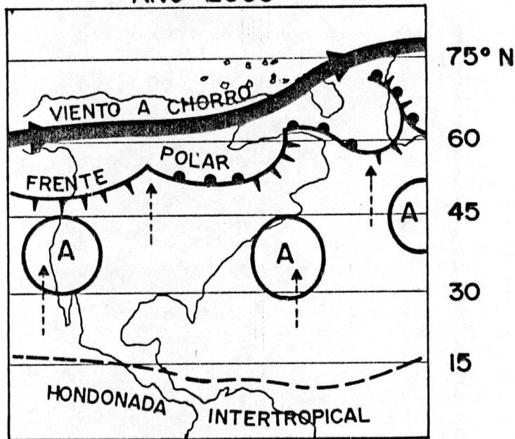
FIG. 15 MODELO SINOPTICO-CLIMATICO AÑO 2035
