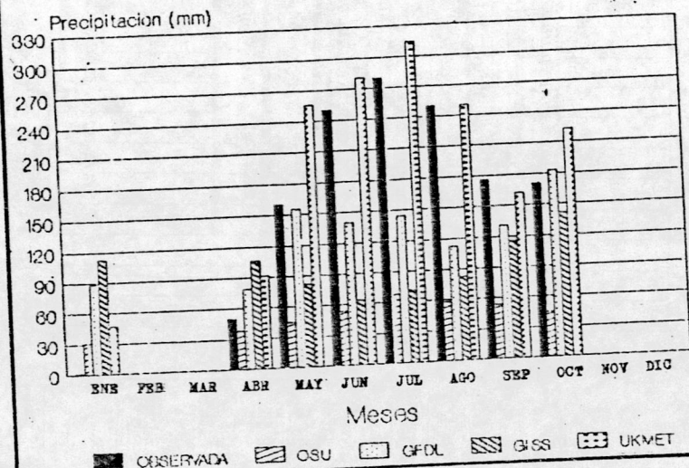
FIG. 3-B COMPARACION ENTRE LA PRECIPITACION OBSERVADA Y LA SIMULADA POR LOS MODELOS OSU, GFDL, BISS Y UKMET CELDA 9- SANTA ELENA (LAT. 4-5 N. LONG. 61-62 W.)
