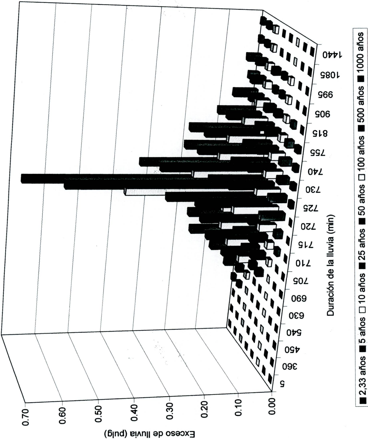
Figura 6. Hietogramas de exceso de lluvia de la estación pluviográfica Maiquetía, estado Vargas, Venezuela.
